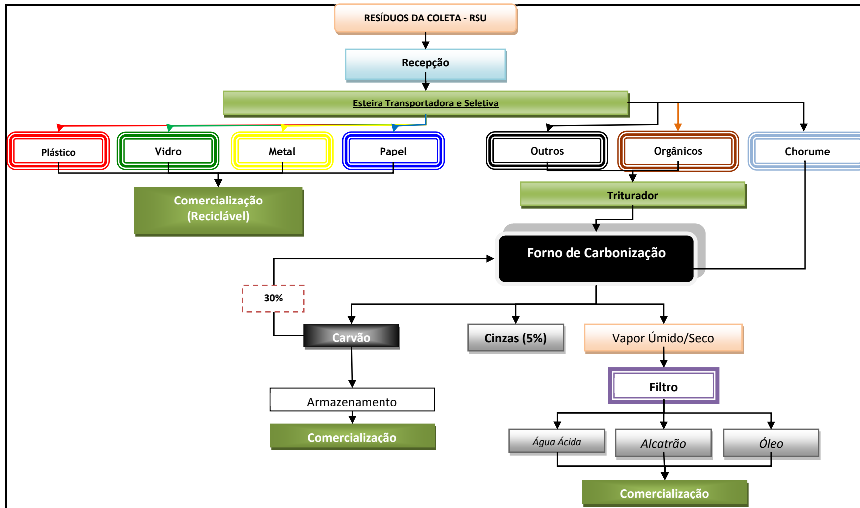
Figura 7: Fluxograma do Processo de Carbonização
