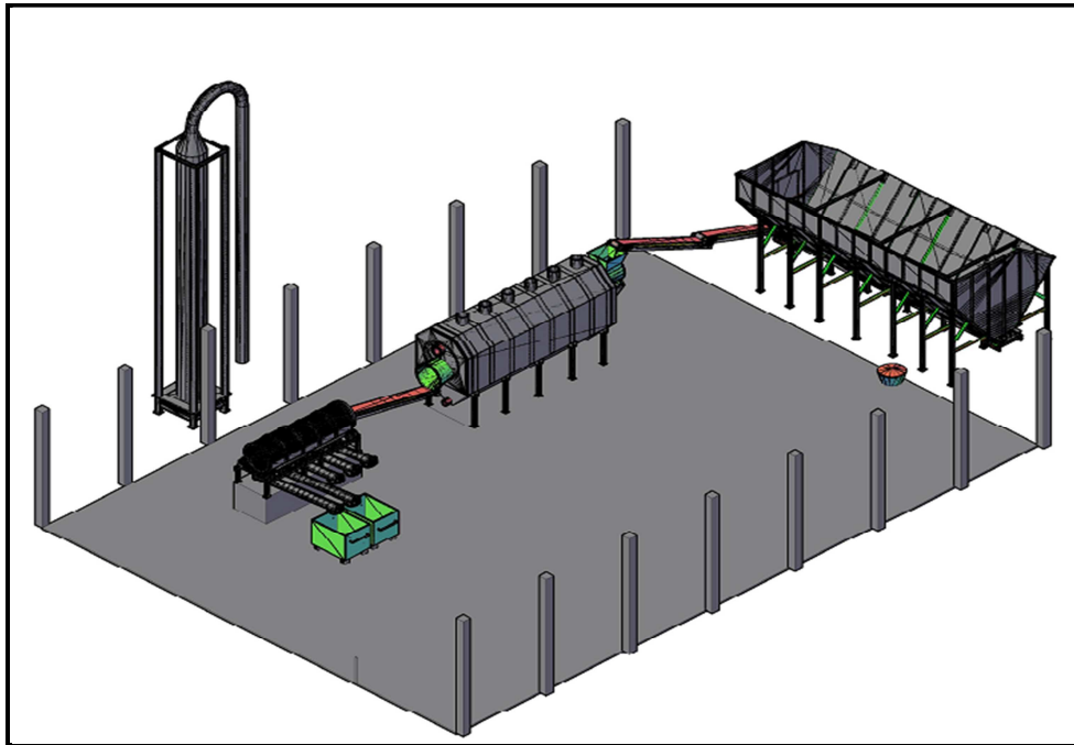
Figura 6: Sistema de Carbonização Montado
